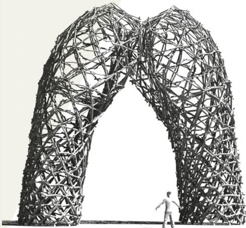
Takto bude vypadat artefakt, který má prověřit plánovanou konstrukci rozhledny.
