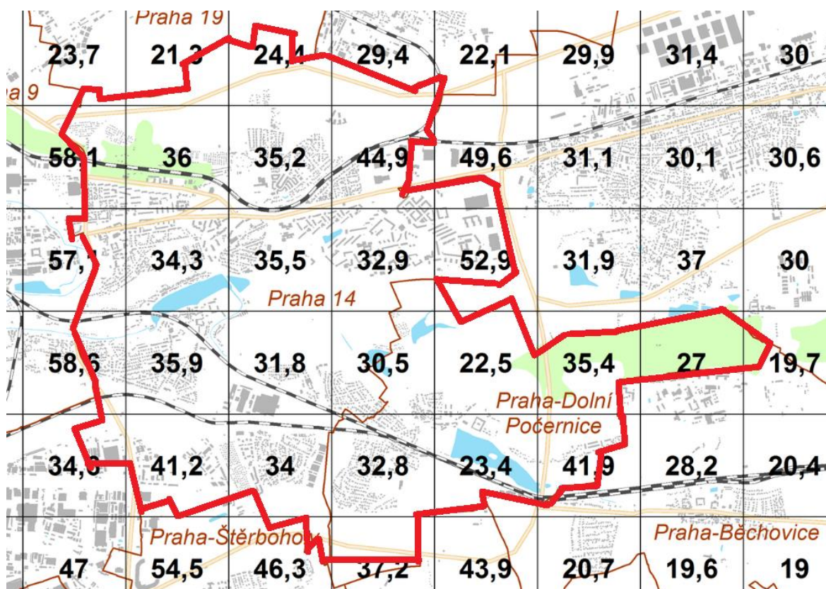
Obrázek 4 - Průměrná koncentrace NO x (Zdroj:ČHMÚ)
