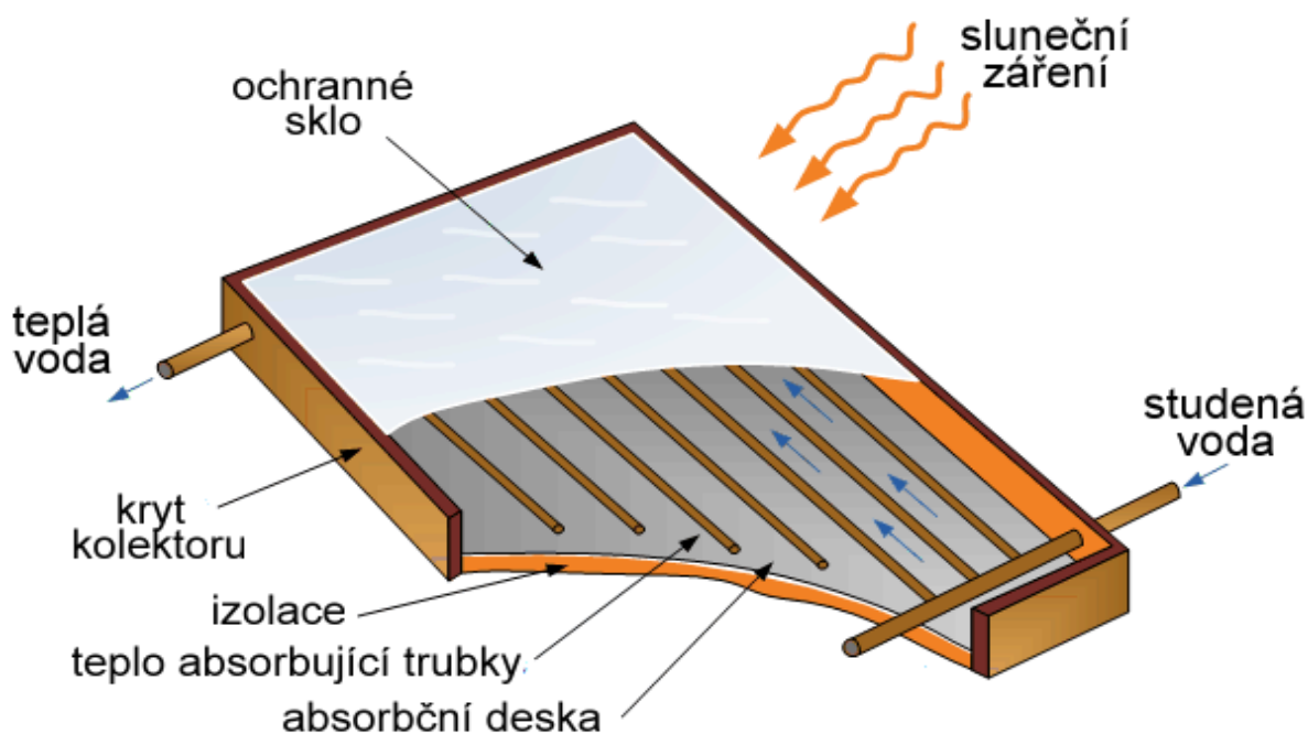
Obrázek 45 Konstrukce plochého kolektoru
