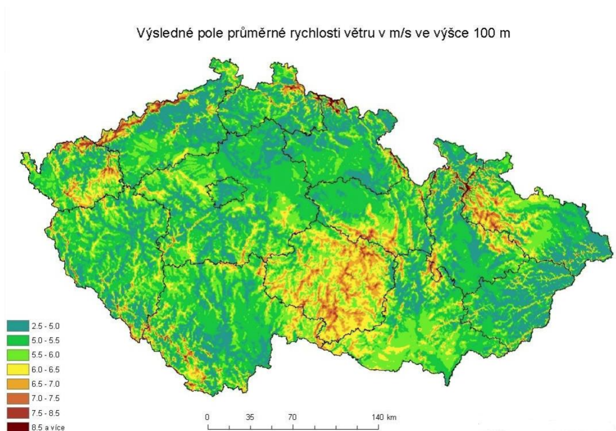
Obrázek 41 Výsledné pole průměrné rychlosti větru v m/s
