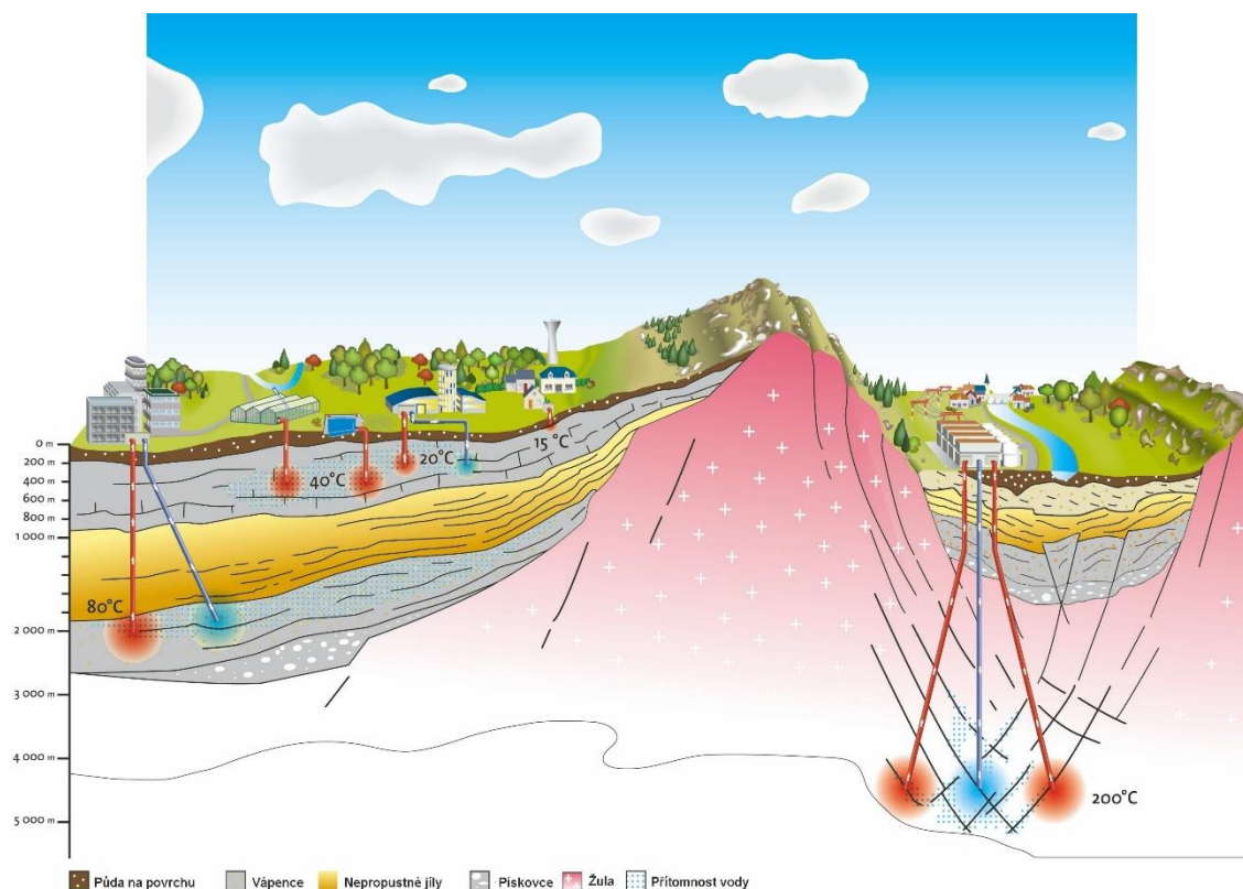
Obrázek 39 - Schéma GTH
